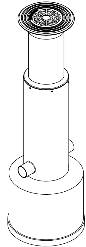
SVK 400/315/170 mittatilauskaivo
